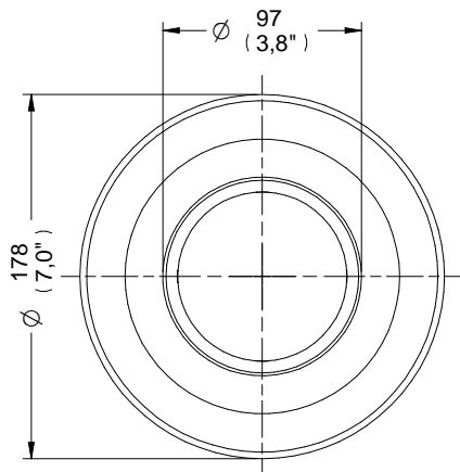
Medidas Referenciales/Estimated Dimensions, Acot.mm.(pulg)/Dim.mm.(in)
