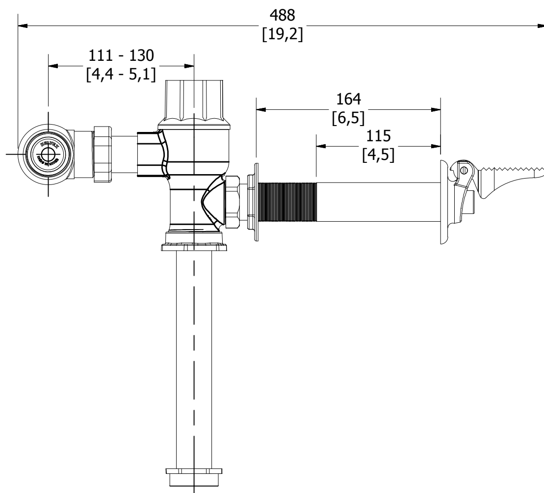
Medidas Referenciales / Estimated Dimensions, Acot.mm.[pulg] / Dim.mm.[in]
