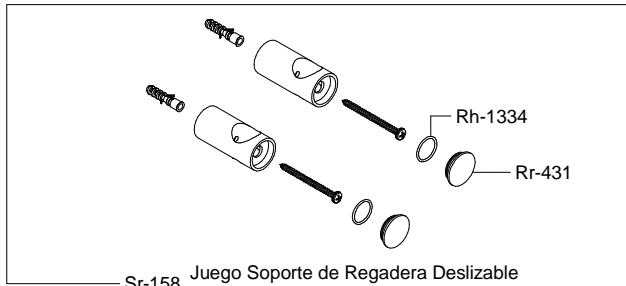
Sr-158 Juego Soporte de Regadera Deslizable Sliding Shower Game Support
