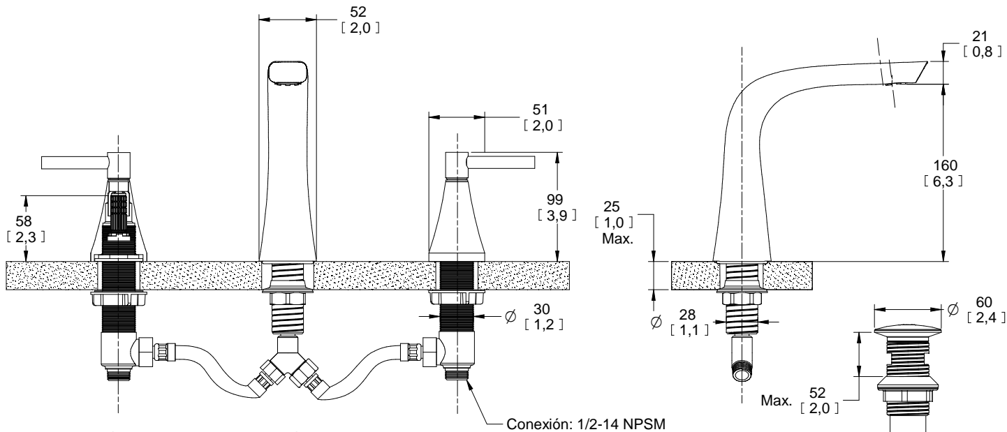
Medidas Referenciales / Estimated Dimensions, Acot. mm [pulg.] / Dim. mm [inch.]
