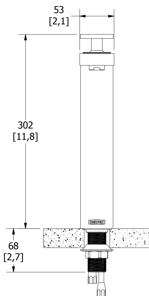
Medidas Referenciales / Estimated Dimensions, Acot. mm [pulg.] / Dim. mm [inch.]
